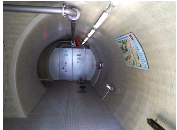
Der neu gebaute Hochbehälter Elmau - eine Glasfasersonderkonstruktion
