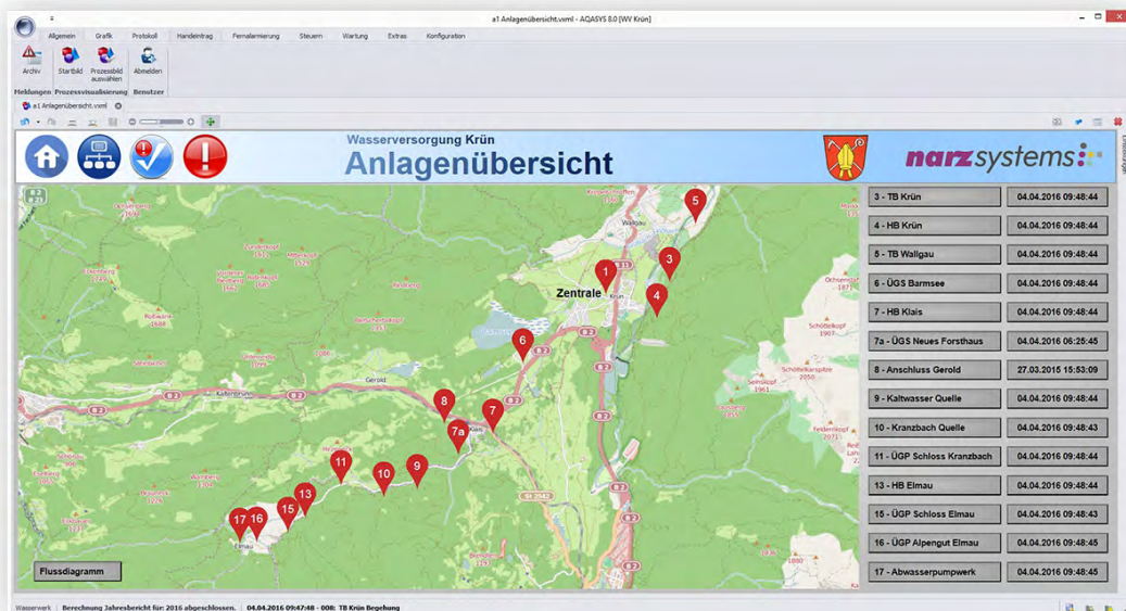
Anlagenübersicht mit topographischer Karte, erstellt mit dem AniMMeX Evolution Prozessbildeditor
