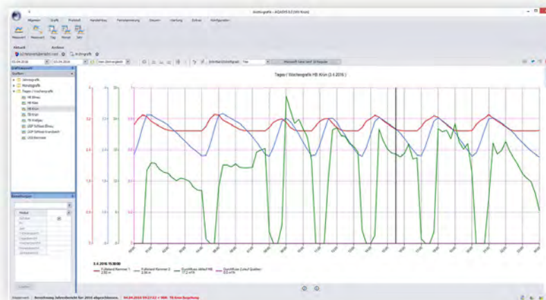
Tagesganglinie des Hochbehälters Krün aus dem AQASYS™ Prozessleitsystem
